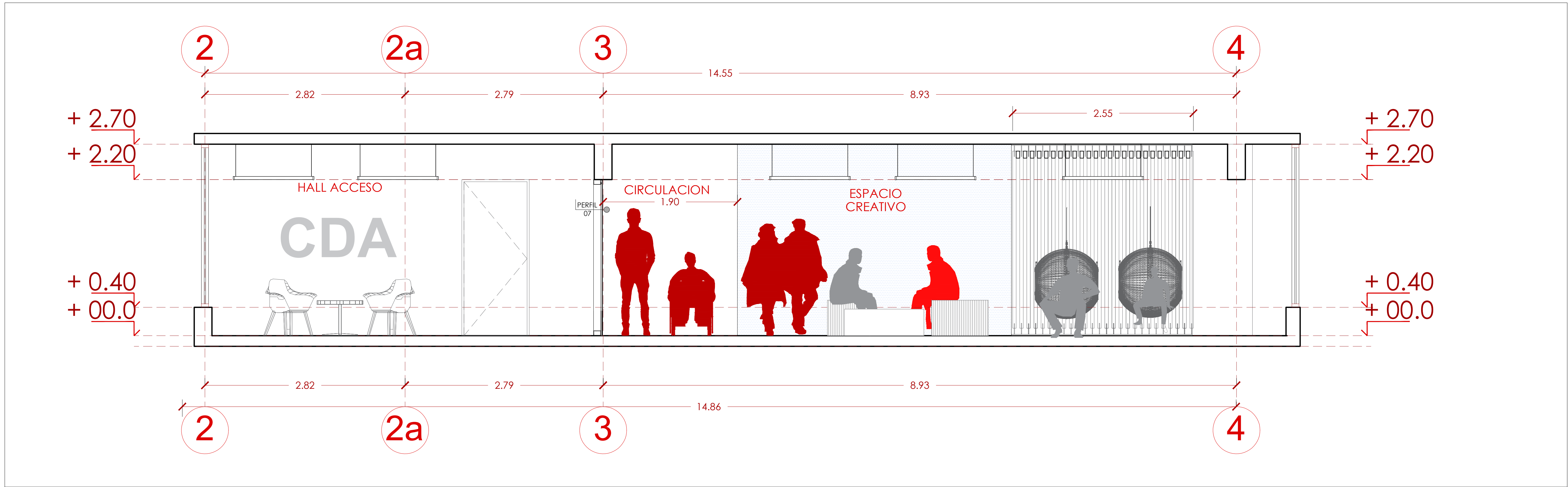
3 CORTE DE AQRUITECTURA B-B Escala: 1:100
