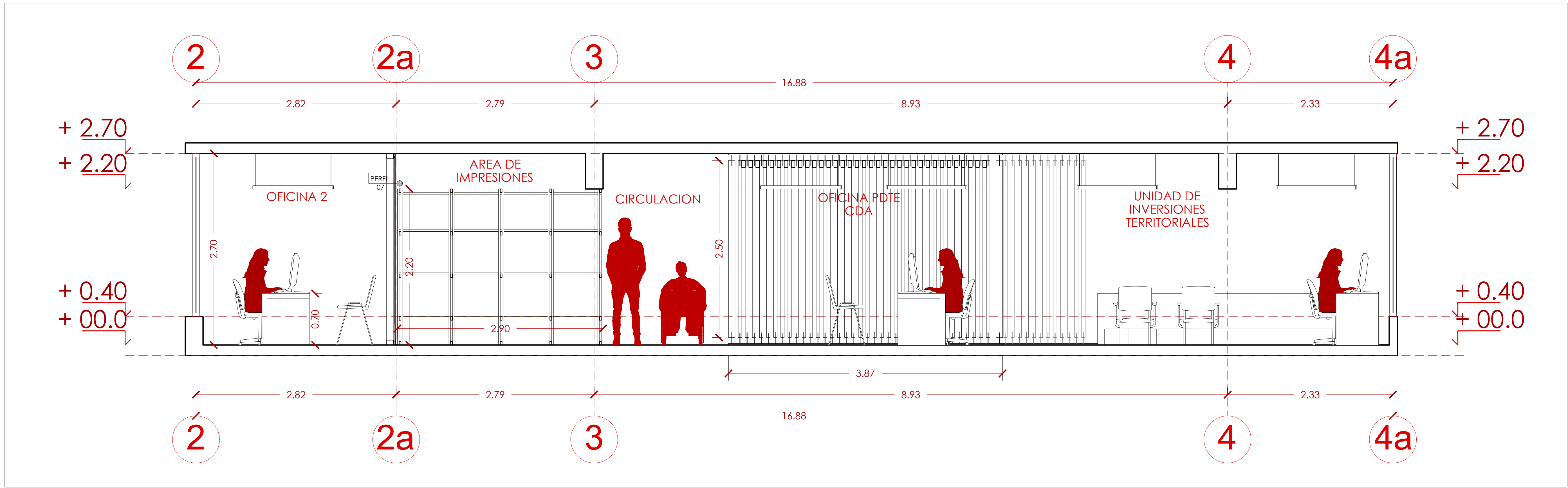
2 CORTE DE ARQUITECTURA A-A Escala: 1:100
